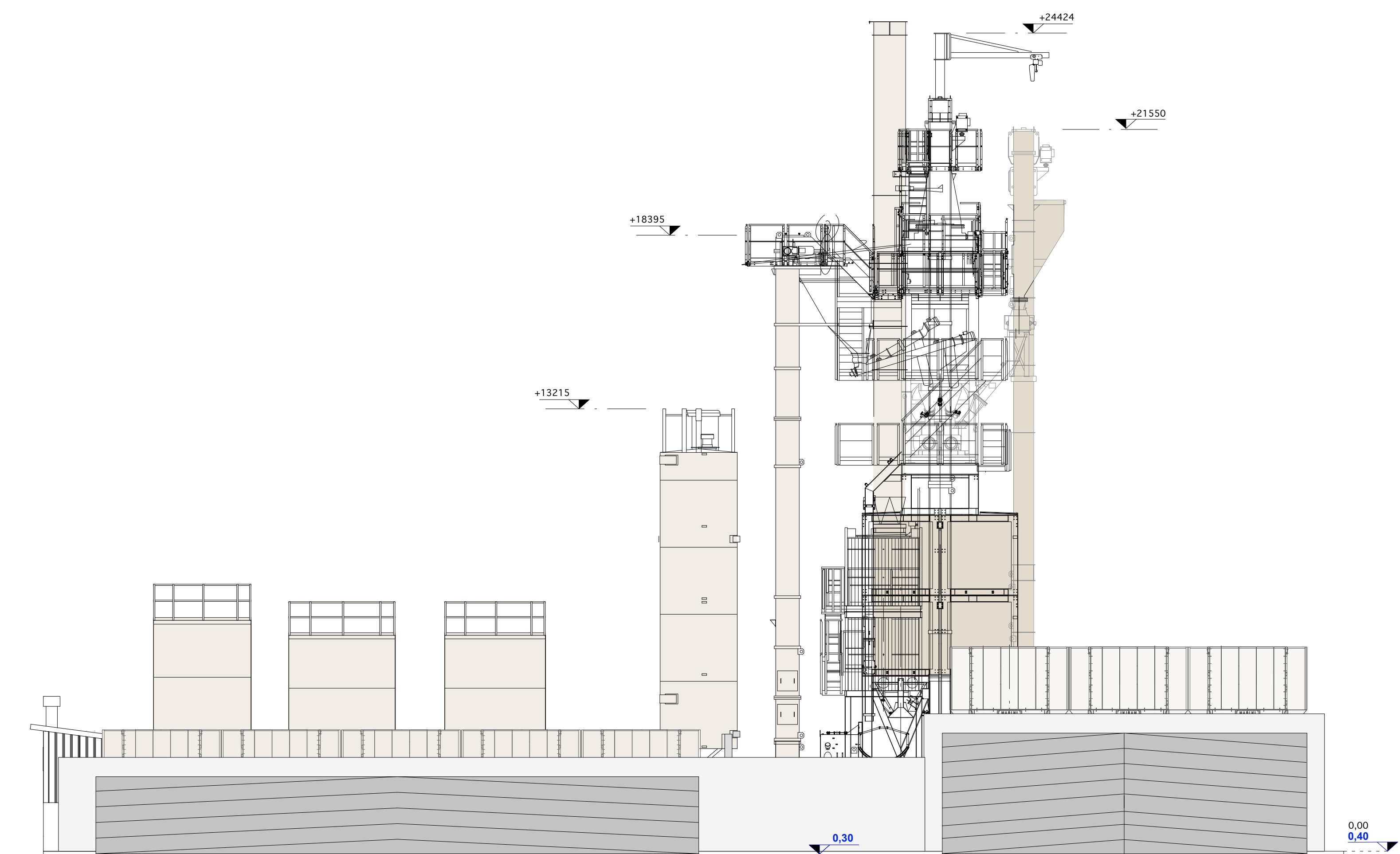
PROSPETTO 02
