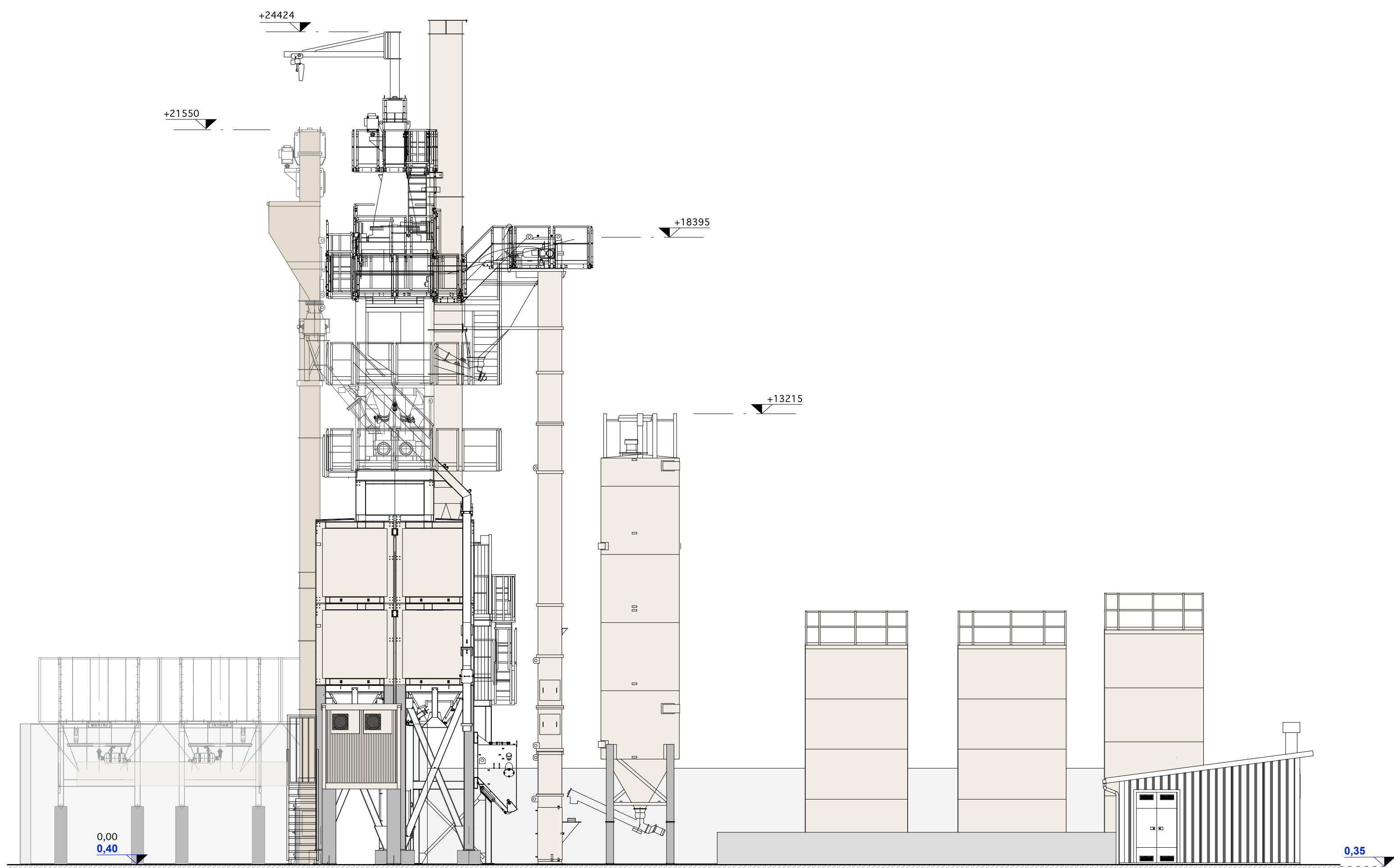
PROSPETTO 02
