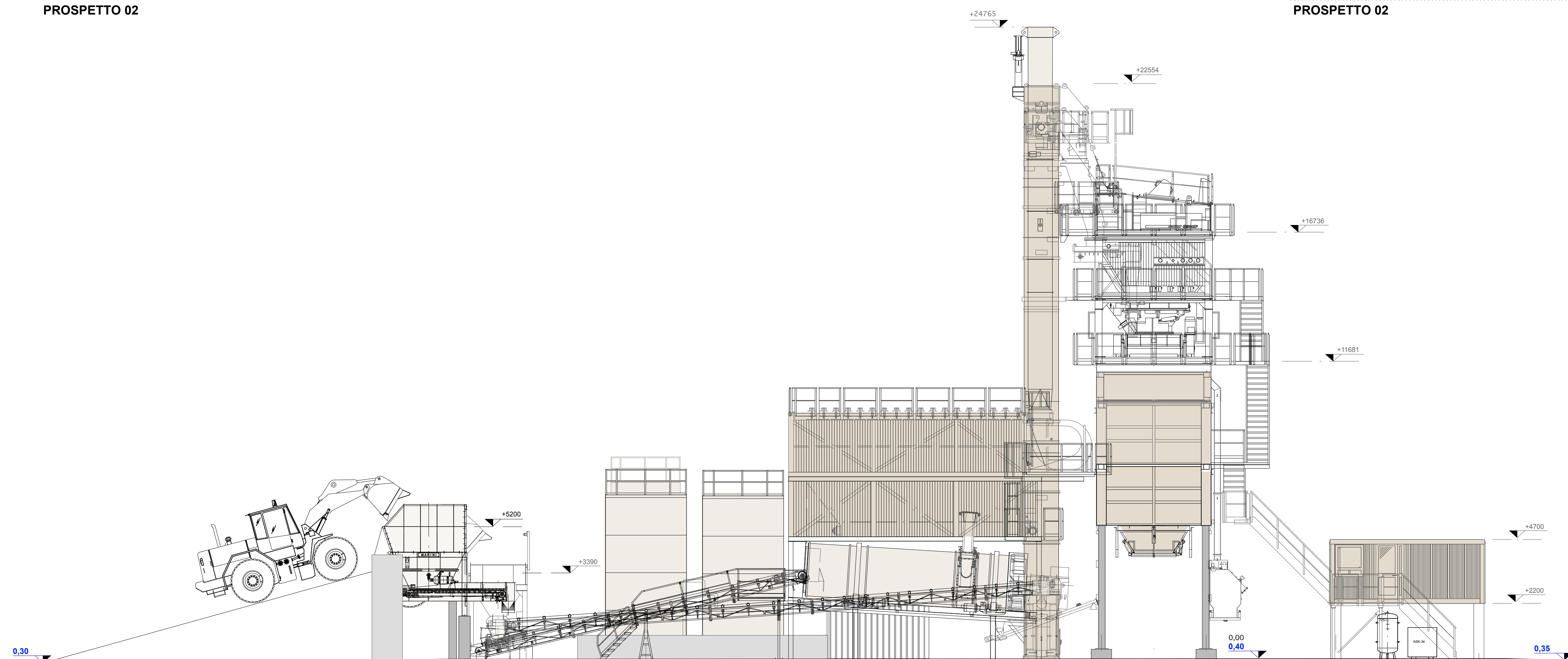
PROSPETTO 03
